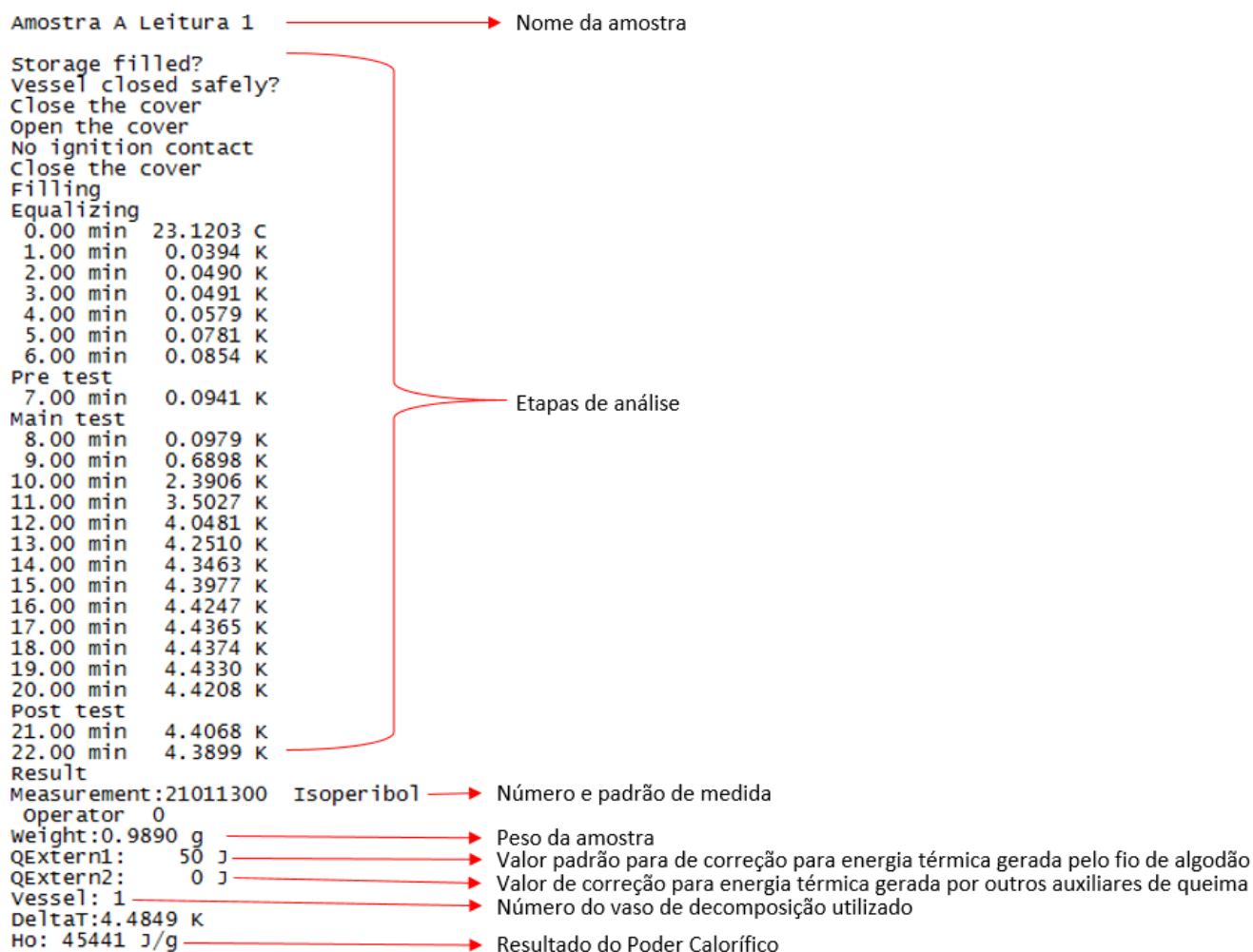
Figura 1: Apresentação dos resultados da bomba calorimétrica Ika, modelo C200.
